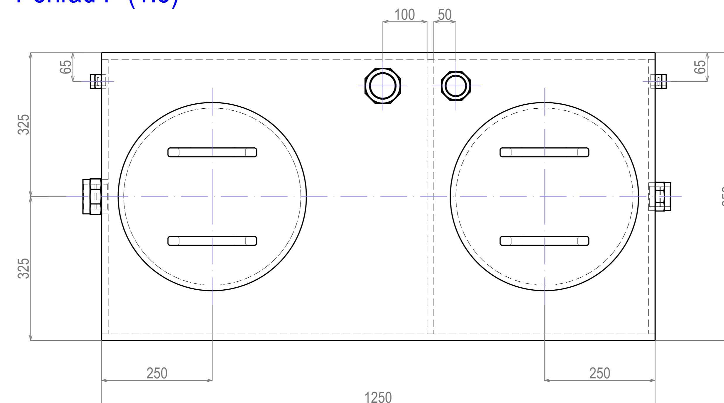
Pohľad P (1:5)
