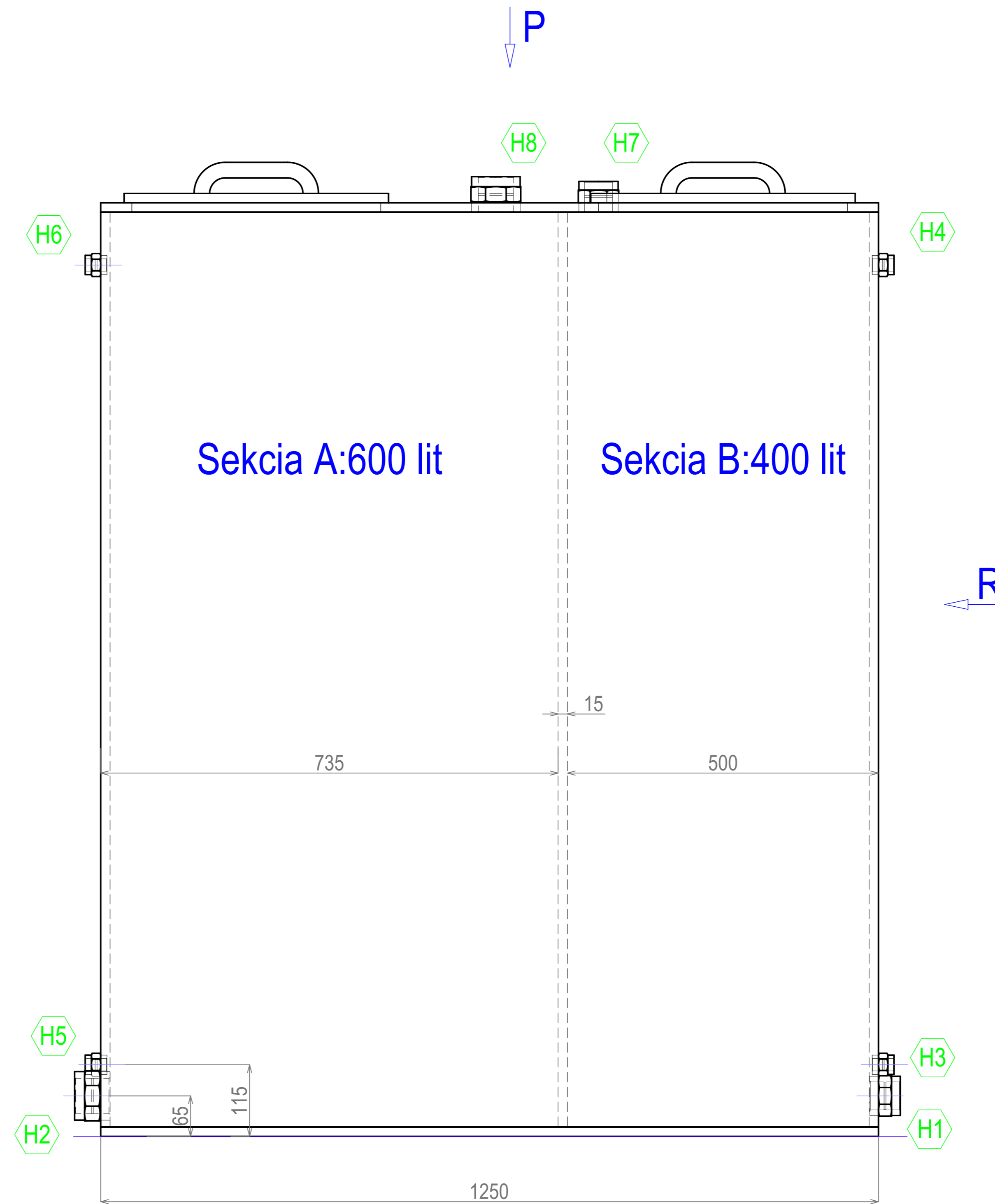
Pohľad P (1:5)
